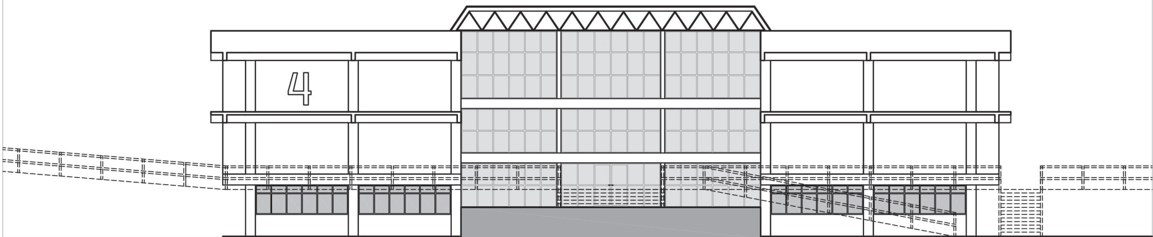
FACHADA OESTE ESCALA 1/200
