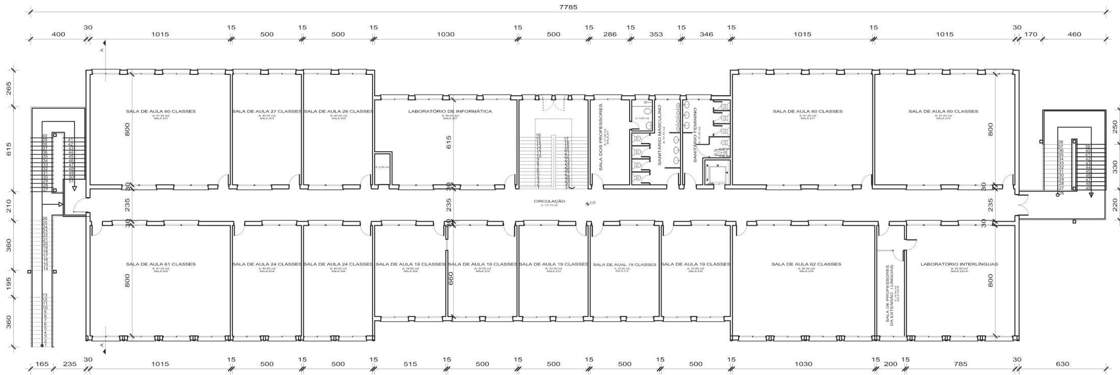
2º PAVIMENTO ESCALA 1/200
